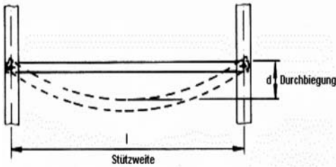
Abb. 1: Höchstzulässige Durchbiegung der tragenden Elemente von Lagereinrichtungen
