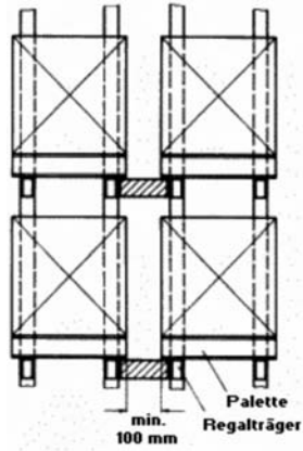
Abb. 8b: Sicherheitsabstand
