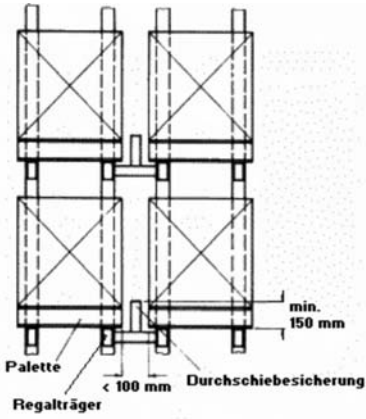
Abb. 8a: Durchschiebesicherung
