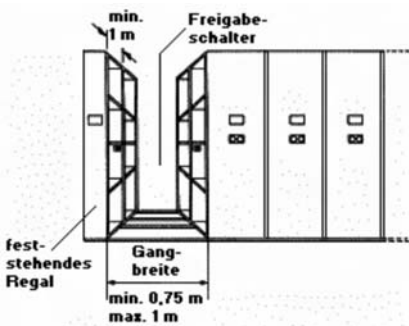
Abb. 16: Sicherung durch Freigabeschalter
